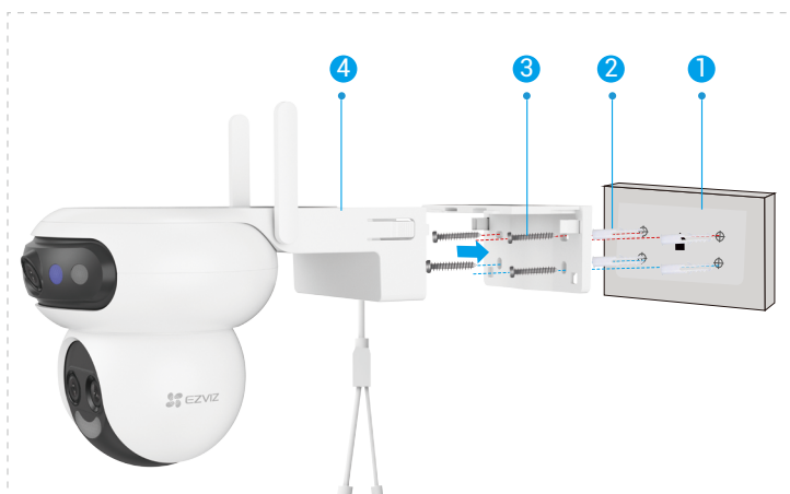
Fig. 2 Montage mural
